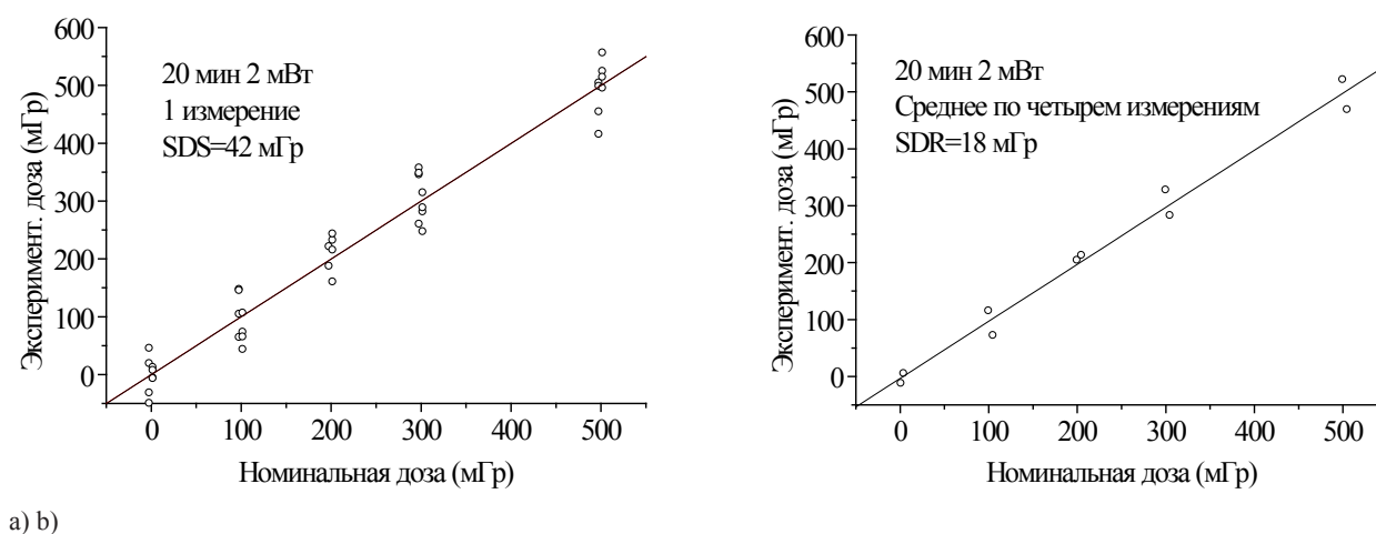
Рисунок 1 – Примеры зависимостей экспериментальных доз от номинальной дозы, при одинарном измерении спектра (а), средние результаты, полученные для четырех повторных измерений спектров (б). Измерения спектров проводят при СВЧ-мощности 2 мВт и времени накопления 20 мин.
