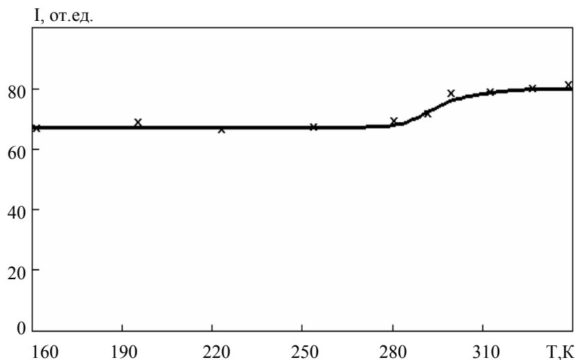
Рис. 5. Температурная зависимость выхода примесной люминесценции у предварительно облученного KPO_3-Tl^+
