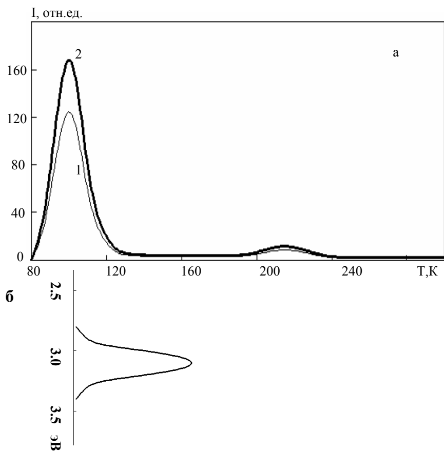
Рис.1. (а) - Кривые ТСЛ метафосфата калия в кристаллическом состоянии. 1 – доза облучения 100 Гр, 2 – 300 Гр. (б) – спектральный состав пика ТСЛ
