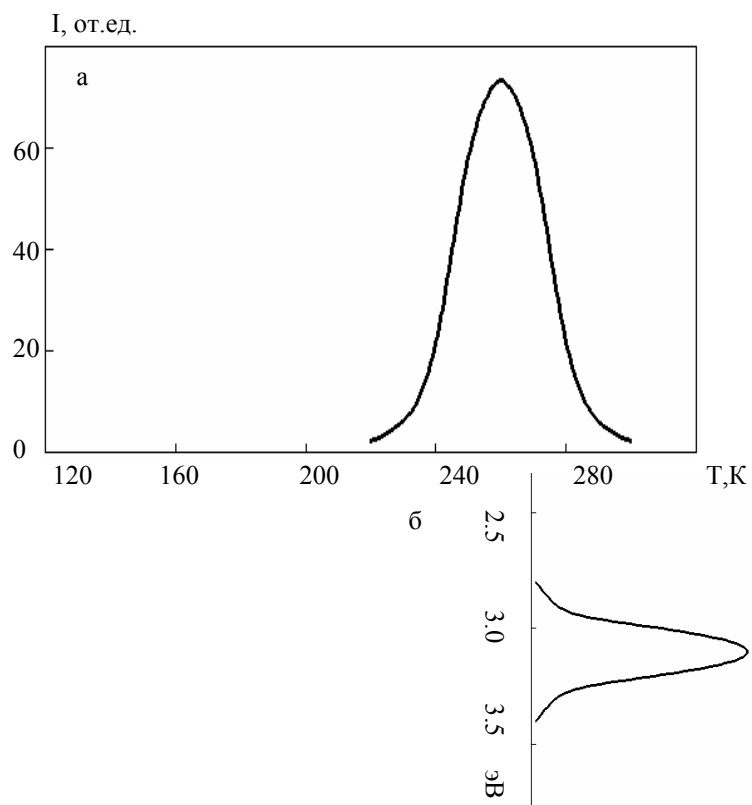
Рис. 2. Кривая ТСЛ (а) и спектральный состав (б) пика ТСЛ для стеклообразного KPO_3 . Доза облучения 500 Гр
