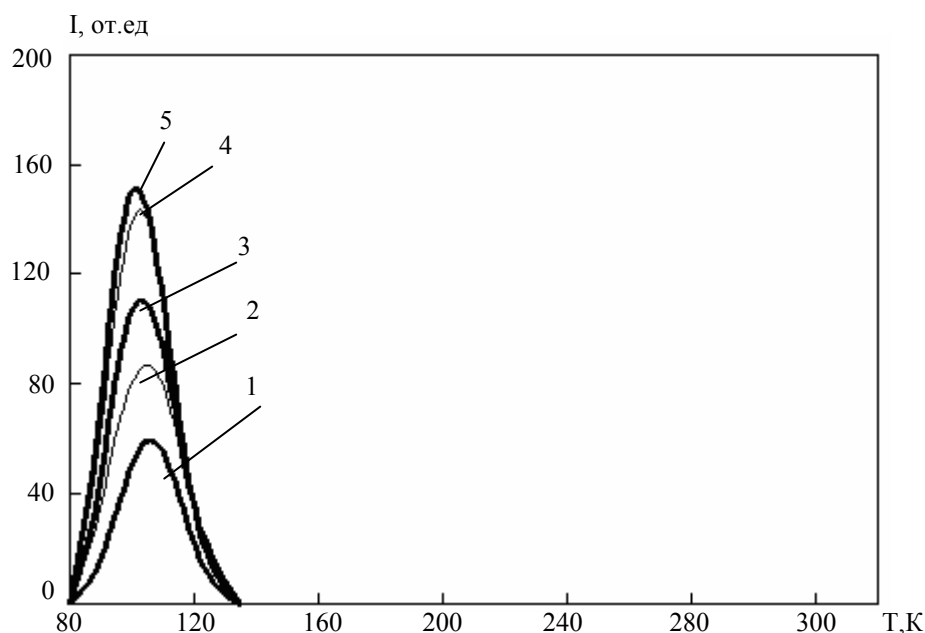
Рис.3. Кривая ТСЛ KDP активированного ионами марганца после предварительного термообработки до 350°С. Дозы облучения – 40 Гр (1), 60 Гр (2), 80 Гр (3), 100 Гр (4), 120 Гр (5)
