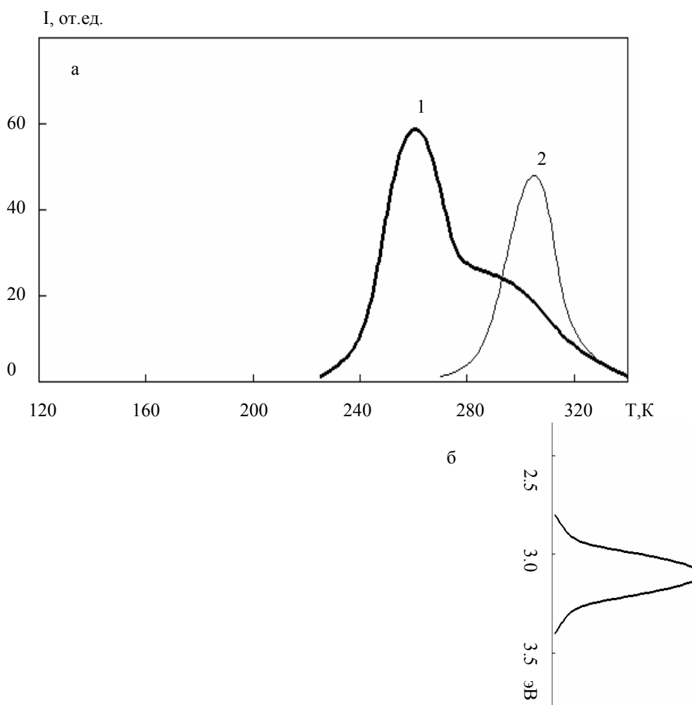
Рис. 4. Кривая ТСЛ (а) и спектральный состав (б) пика ТСЛ для кристалла \text{KPO}_3\text{-Tl}^+ . Доза облучения 0.5 кГр
