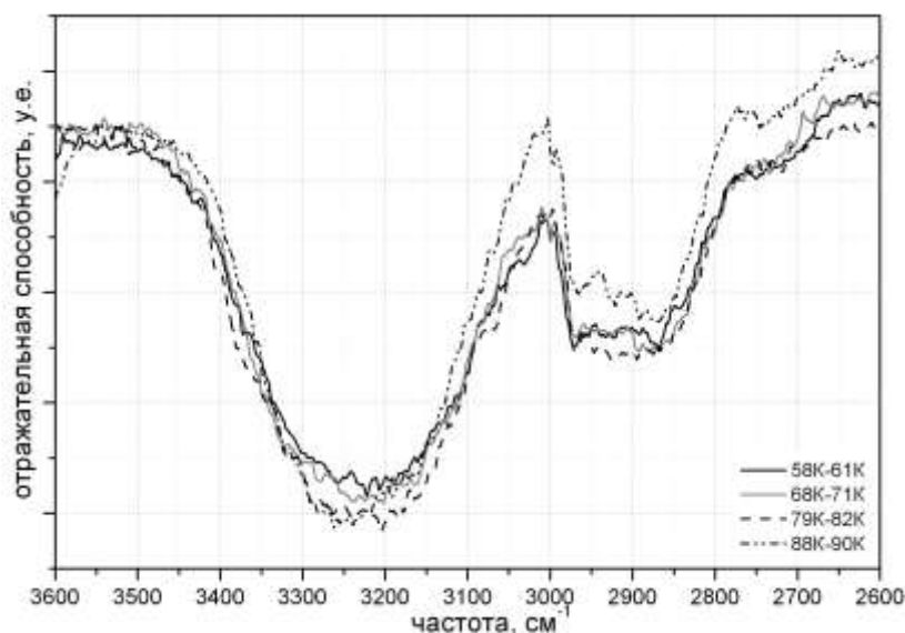
Рис. 3. ИК-спектры в диапазоне характерных колебаний О-Н и С-Н связей, пленки твердого этанола в различных структурных состояниях при температурах 58-90К. Толщина пленки d=0,75 мкм, температура конденсации T=16 К. Скорость отогрева V_{\text{анн.}} \approx 0.01 К/с
