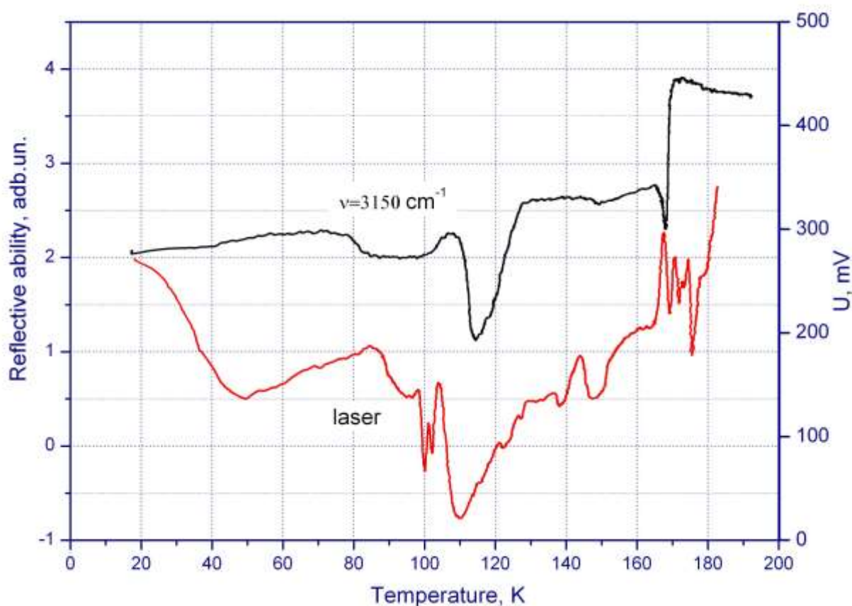
Рисунок 1 – изменения сигналов спектрометра при частоте 3150\text{ cm}^{-1} и лазерного интерферометра в процессе отогрева пленки криоконденсата этанола. Скорость нагревания 2\text{ K/min} , толщина пленки d=2\text{ }\mu\text{m} .
