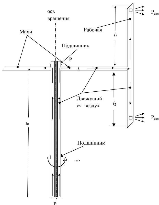
Рисунок 2 – Естественная вентиляция воздуха, вследствие работы центробежных сил
