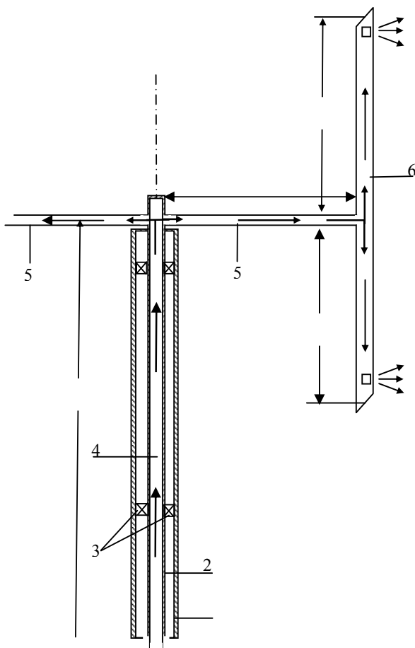
Рисунок 5 – Принципиальная конструктивная схема турбины типа Н – ротор
