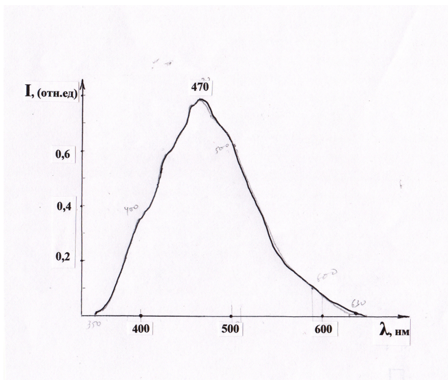
Рисунок 2 – Спектр фотолюминесценции пористого алюминия
