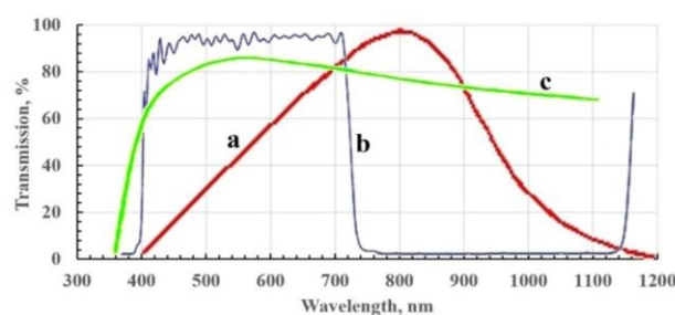
Рисунок 1 – В обоснование повышения чувствительности цифровых камер в ближней инфракрасной области
