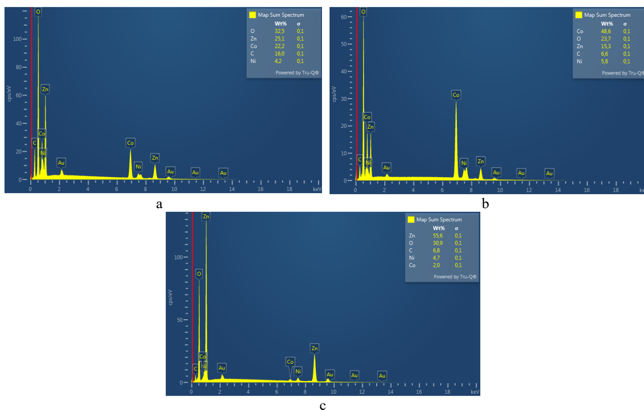
Рисунок 2 – EDS спектры: (а) образец #2, (b) образец #4 и (с) образец #6
