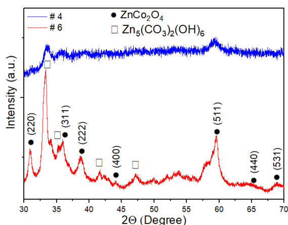
Рисунок 3 – XRD анализ образцов \text{ZnCo}_2\text{O}_4 #4 и #6
