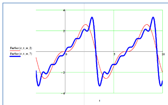
10-сурет. \varepsilon(t) = t функциясының графиттік шешімі
