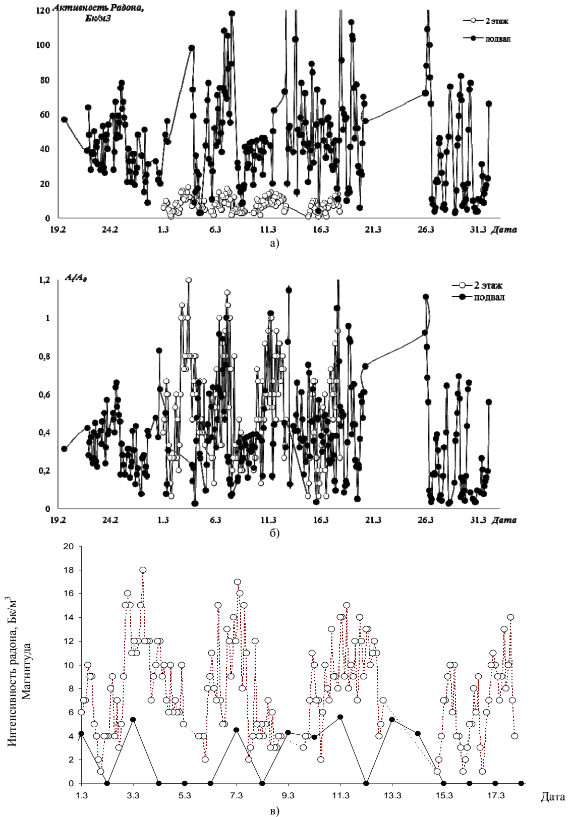
а) в реальном масштабе; б) в относительных единицах для измерений на высотах: – 3м (подвал), + 6 м (2 этаж); в) корреляция эманации радона (светлые точки) с магнитудами землетрясений (темные точки)
