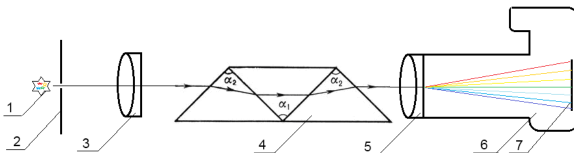
1 – источник; 2 – микрометрическая щель; 3 – объектив; 4 – призма Амичи; 5 – объектив фотоаппарата; 6 – цифровой фотоаппарат; 7 – матрица.
